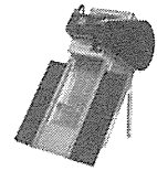
スクリーン
